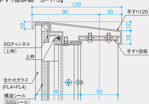
【手すり部詳細 S=1/3】
