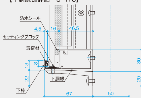
【下胴縁部詳細 S=1/3】
